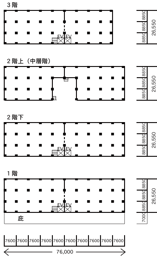
倉庫平面図
