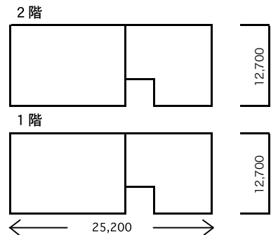
事務棟平面図
