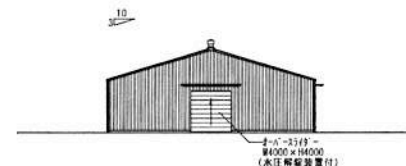
東側立面図
