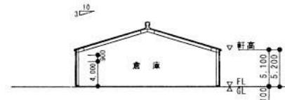
断面図
