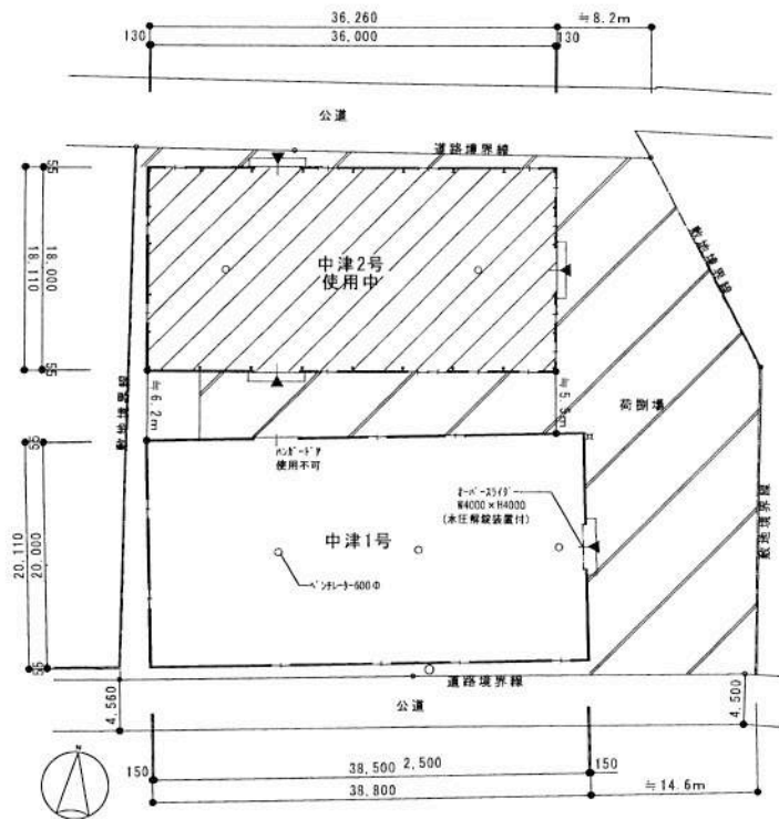
配置・平面図
